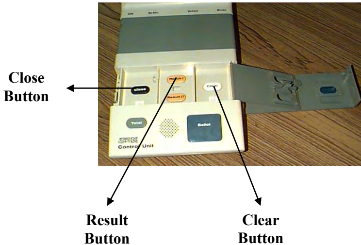
Fig. 10.10: “Result” Sections
